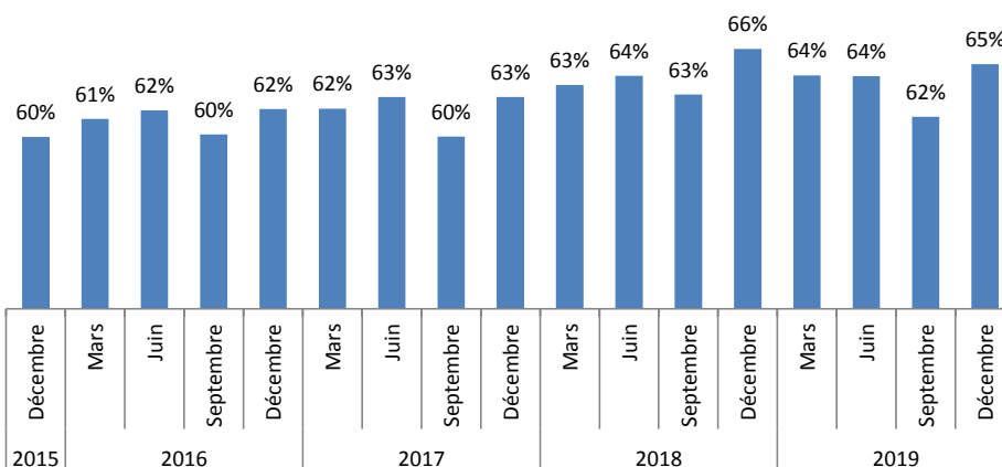
Evolution de la part des DEFM indemnissables inscrits (cat ABC) - Bagnols sur Cèze
